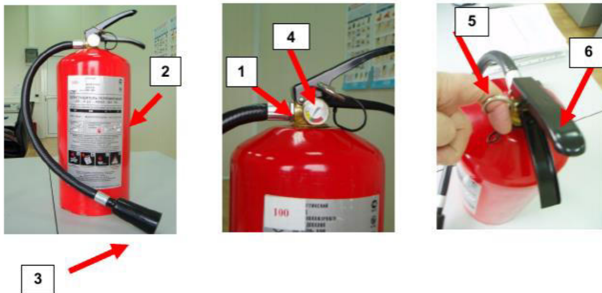
Рисунок 4 - Порошковый огнетушитель типа ОП-4(з)
