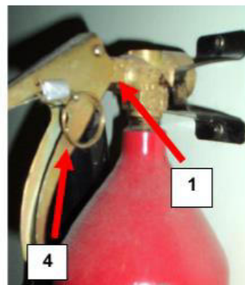
Рисунок 5 - Углекислотный огнетушитель типа ОУ-3
